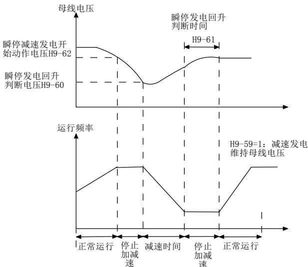
图 6-21 瞬时停电动作示意图
