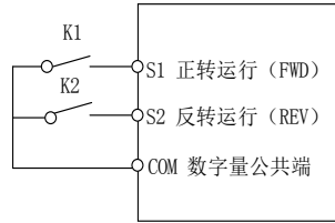
图 6-3 两线式模式 1
